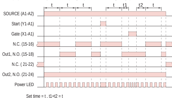
輸出模式 B3 ：閃爍反動作(ON先計時)
