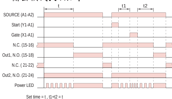
輸出模式 B ：閃爍(OFF先計時)
