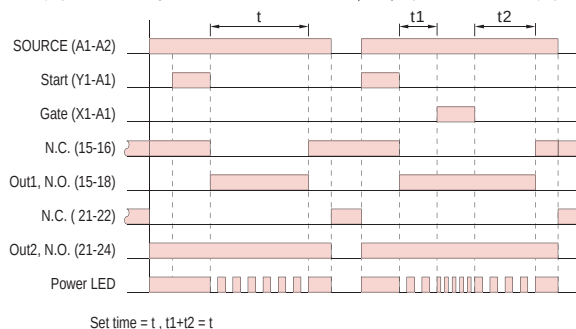
輸出模式 E ：反動作(信號ON計時)
