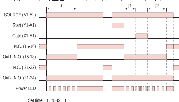
輸出模式 E1 ：反動作(信號OFF計時)
