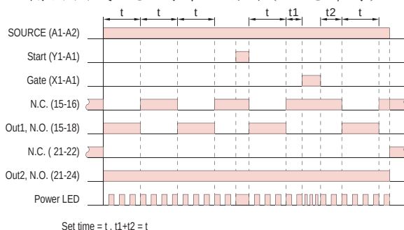
輸出模式 C ：信號ON-OFF計時
