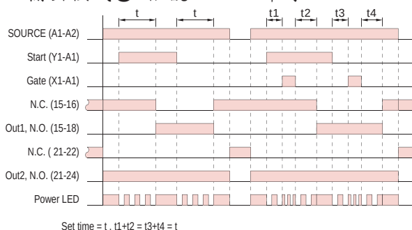
輸出模式 C ：信號ON-OFF計時
