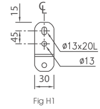
高壓端子圖 H.V. terminal
