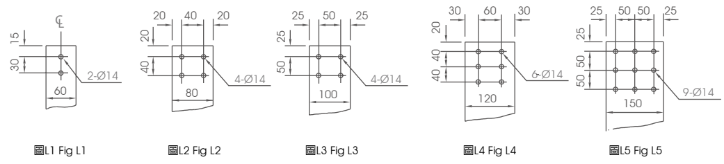
低壓端子圖 L.V. terminal
