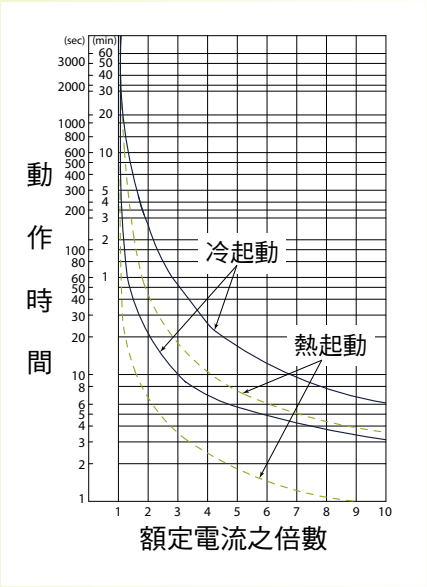
TH-P38N(11A以下) 動作特性曲線
