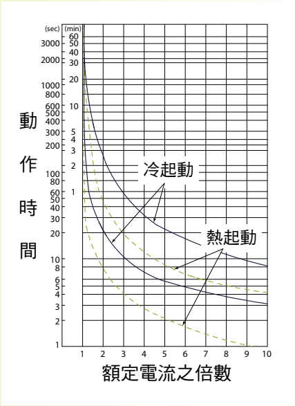
TH-P38N(15A以上) 動作特性曲線
