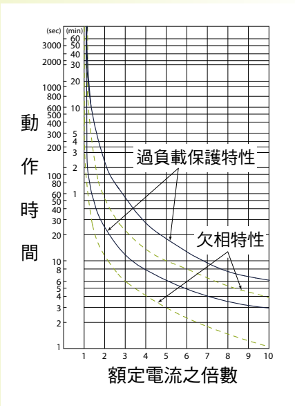
TH-P38NPP 動作特性曲線
