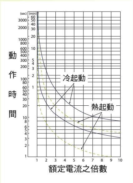
TH-P65N(L) 動作特性曲線
