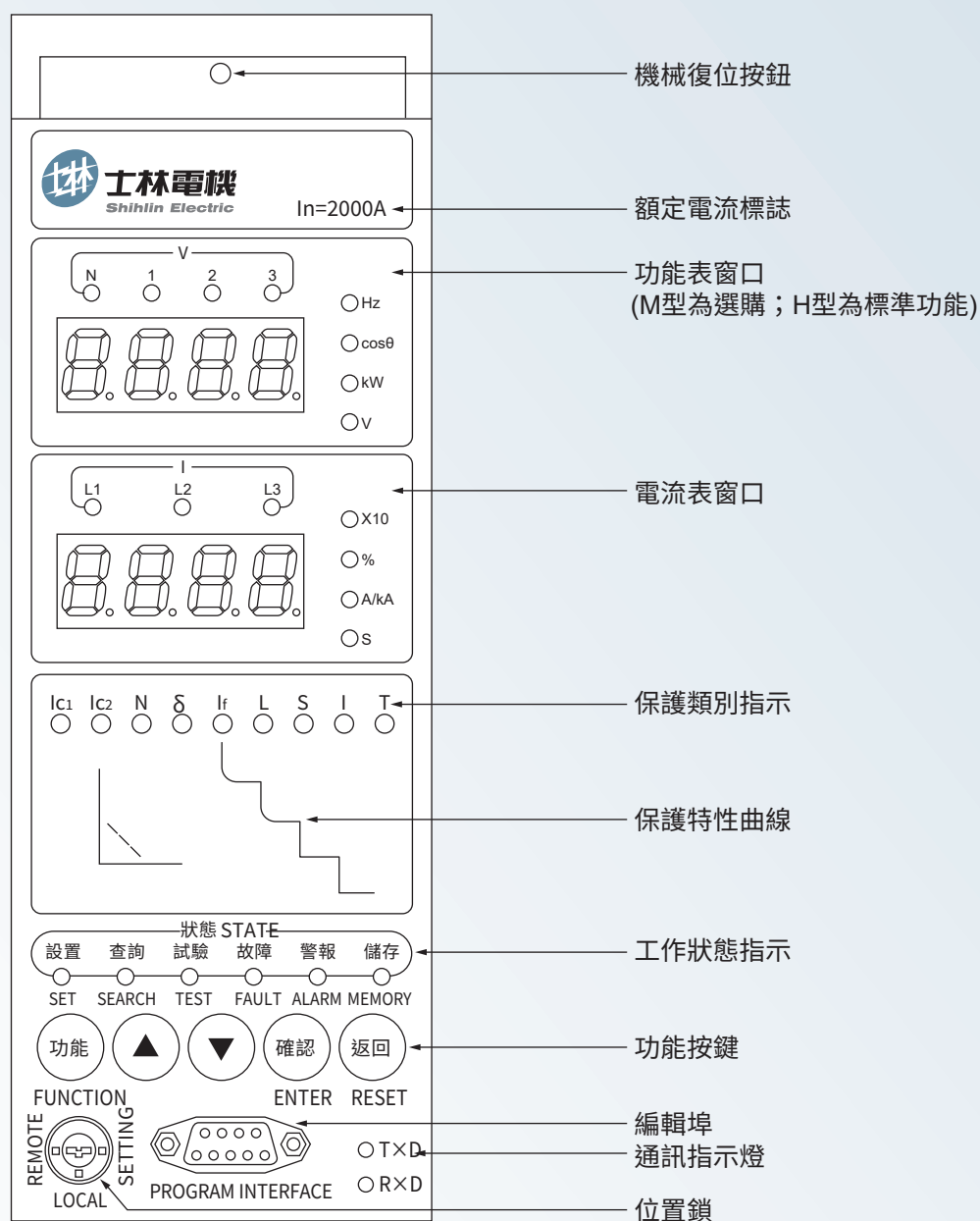
控制器面版
