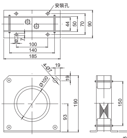
b. ZT100環形互感器尺寸圖
