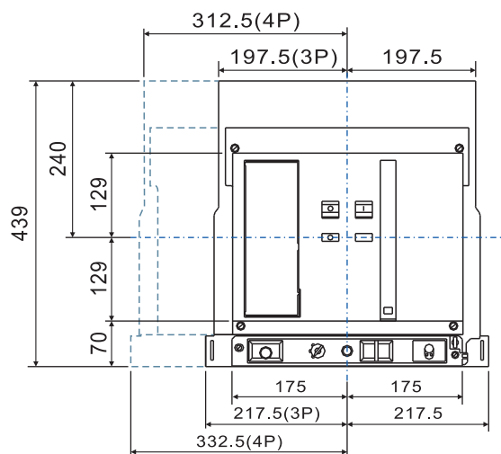
(4) BA3200-H抽出式
