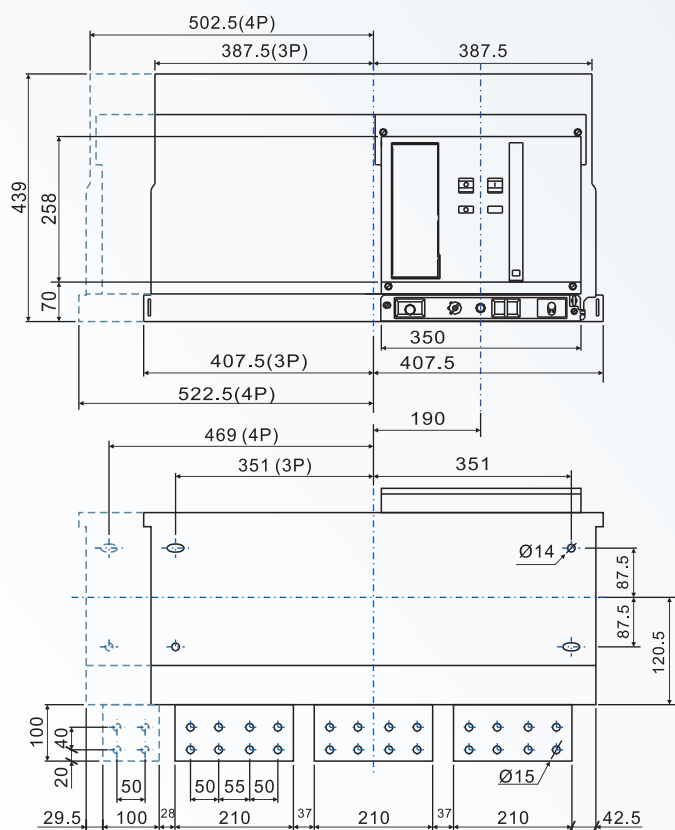
(6) BA5000-H抽出式
