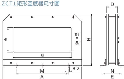
互感器尺寸圖
