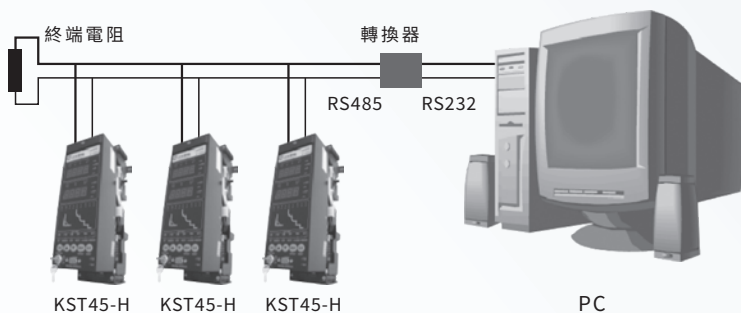
Modbus通信協議接線示意圖
