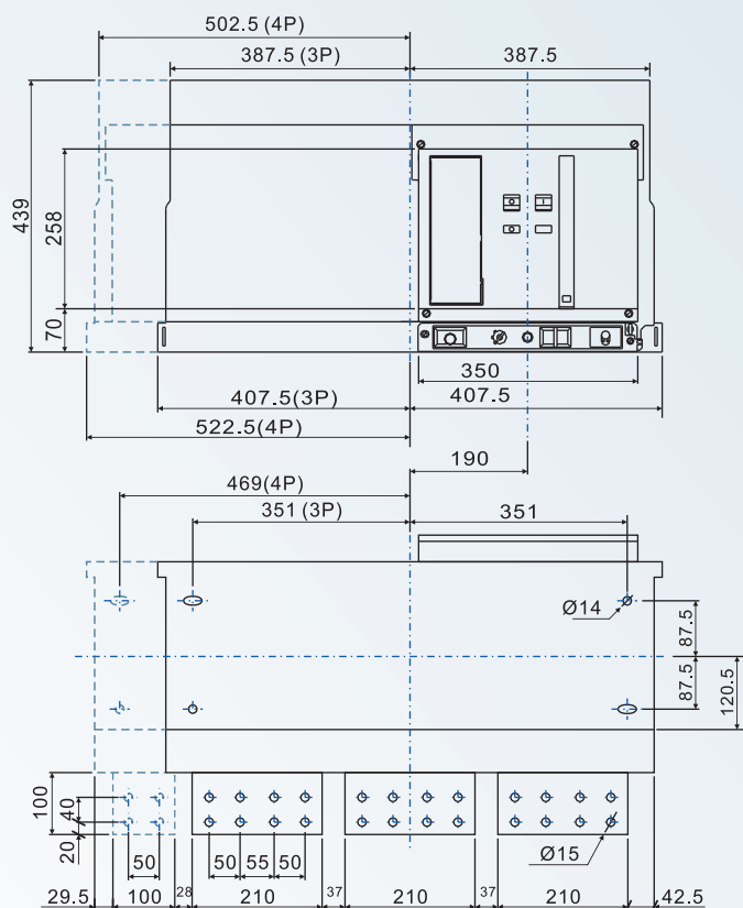
(5) BA4000-H抽出式
