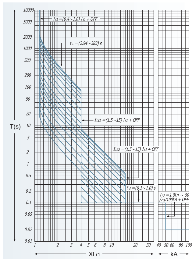
(4) 特快反時限1(馬達保護) T=2.95t \times \ln(N^2/(N^2-1.15))
