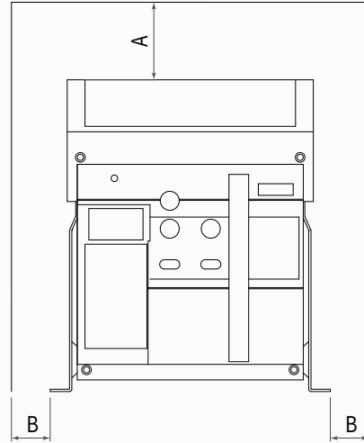
固定式斷路器
