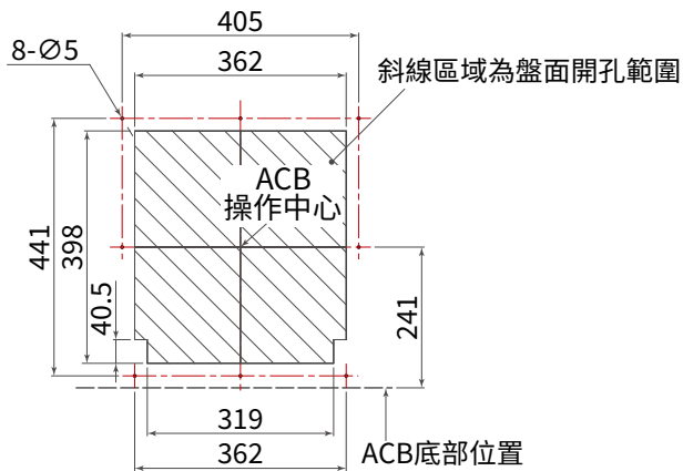
配電盤門及門框(選配)開孔尺寸
