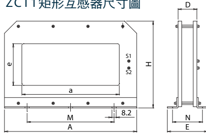
a. ZCT1矩形互感器尺寸圖
