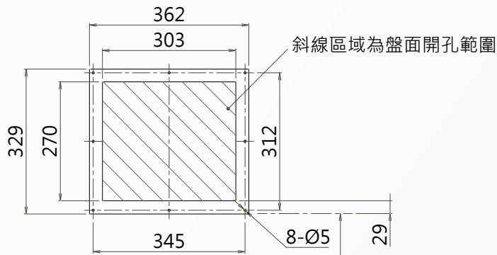
配電盤門及門框(選購) 開孔尺寸 ACB底部位置
